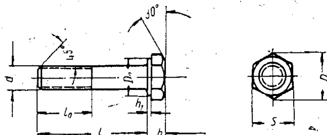
Болт с подголовком
