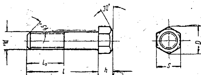
Болт с шестигранной пониженной головкой
