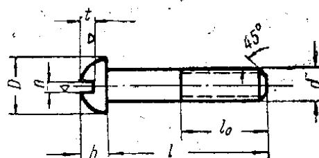
Винт для металла с полукруглой головкой
